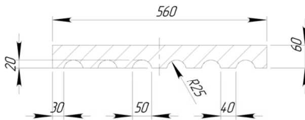
F-F (1 : 10)
