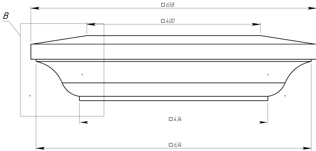
DETA SCALE 1 : 2
